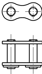
Verschlussglied mit Sicherungsring (DIN 471)
