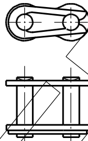
Verschlussglied mit Federverschluss
