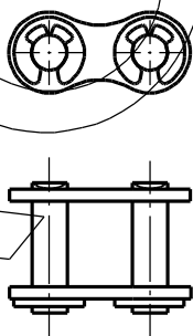
Verschlussglied mit Sicherungsscheibe (DIN 6799)
