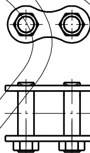
Verschlussglied mit Mutter
